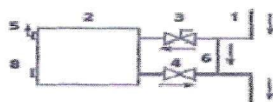
б - однотрубная система, подключение с перемычкой
