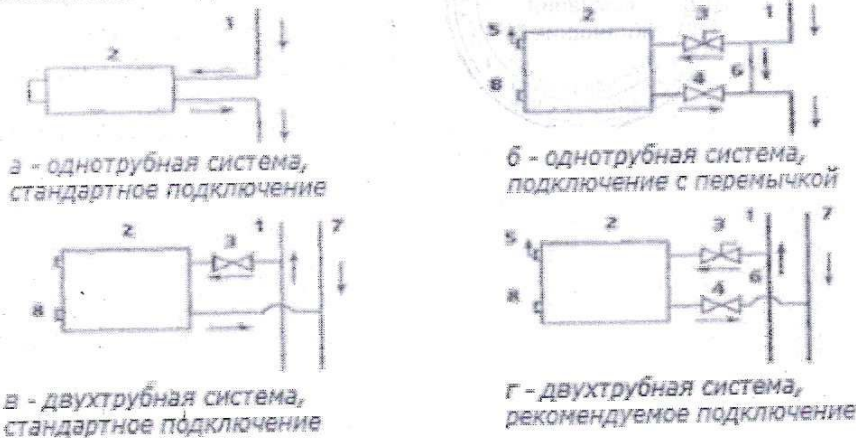
Рис. 1. Цифрами на рисунке обозначены: 1 - падающий стояк, 2 радиатор, 3 - терморегулятор (ручной или автоматический), 4 - вентиль нижний, 5 - воздухоотводчик (ручной или автоматический), 6 - перемычка (байпас), 7 - обратный стояк, 8 - заглушка.
