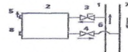
г - двухтрубная система, рекомендуемое подключение
