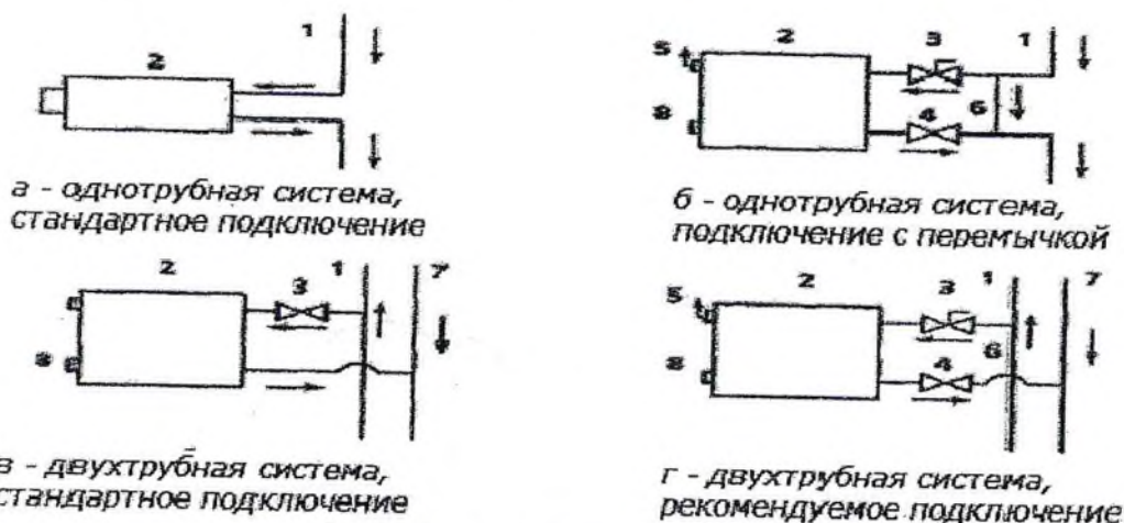
Рис. 1. Цифрами на рисунке обозначены: 1 - падающий стояк, 2 радиатор, 3 - терморегулятор (ручной или автоматический), 4 - вентиль нижний, 5 - воздухоотводчик (ручной или автоматический), 6 - перемычка (байпас), 7 - обратный стояк, 8 - заглушка.
