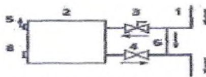
б - однотрубная система, подключение с перемычкой
