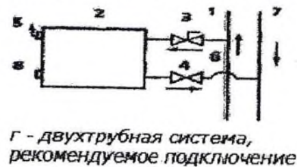
Рис. 1. Цифрами на рисунке обозначены: 1 - падающий стояк, 2 радиатор, 3 - терморегулятор (ручной или автоматический), 4 - вентиль нижний, 5 - воздухоотводчик (ручной или автоматический), 6 - перемычка (байпас), 7 - обратный стояк, 8 - заглушка.
