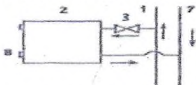
в - двухтрубная система, стандартное подключение
